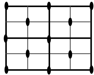
(9) cmm2
