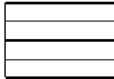
(5) cm
