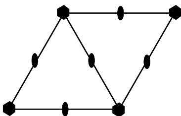
(16) p6
