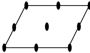
(2) p2
