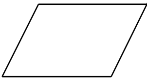
(1) p1
