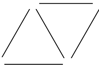
(13) p3
