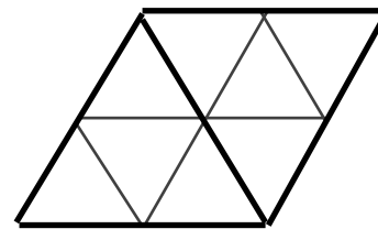
(15) p31m
