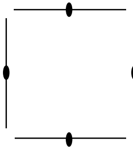
(10) p4
