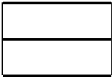
(3) pm
