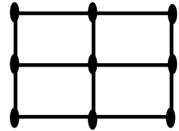
(6) pmm2
