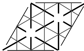
(14) p3m1
